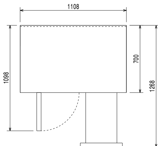
Boven aanzicht
